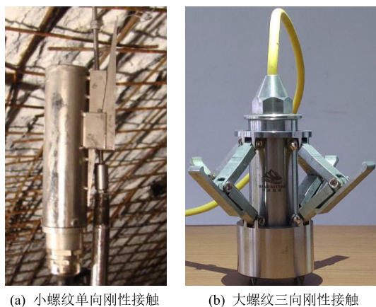
图 1 传感器快速安装与回收装置
