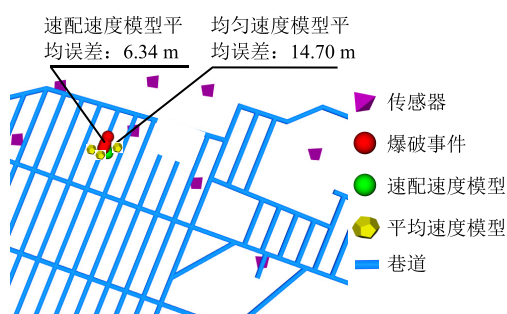
图 7 基于均匀速度模型和数据库动态速配速度模型爆破事件定位结果对比图
